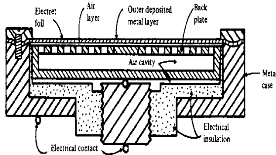
شکل شماره 3- نمایی از ساختار میکروفن الکترو
